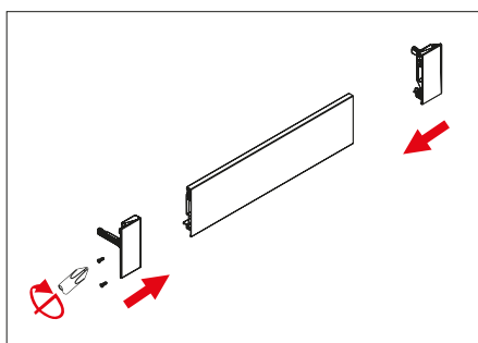
Montaža ličnice notranjega predala
