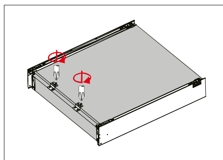
Pri širinah nad 400mm sta priporočena dva pritrdilca
