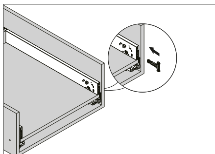
Vstavite šablone v stranici
