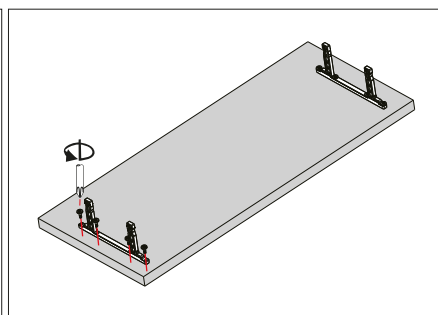
Privijajte pritrdilce ličnic
