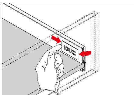
Demontaža ličnice in snemanje predala
