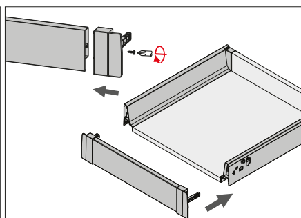
Montaža slepe ličnice
