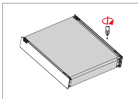
Pritrjevanje dna
